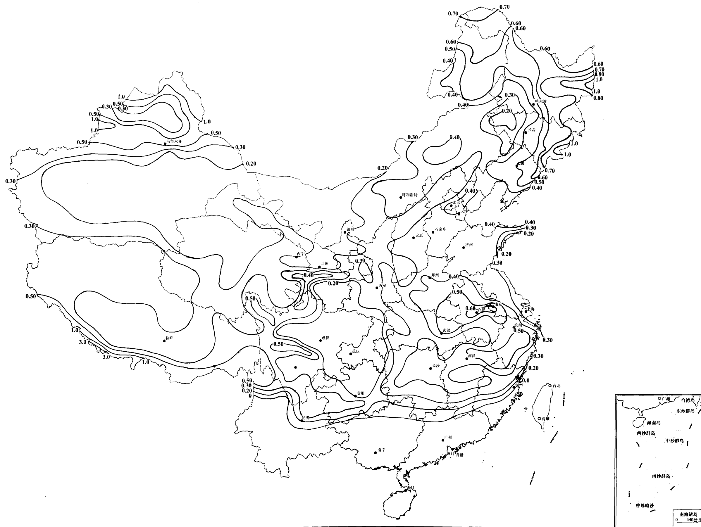
图 E. 6. 1 全国基本雪压分布图( \text{kN/m}^2 )
