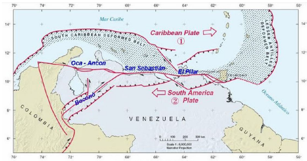
Figura 4.19: Esquema de límites de placas para Venezuela
