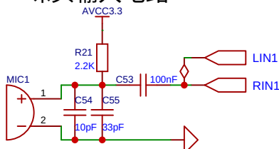
咪头输入电路
