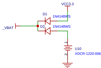
后背电源
