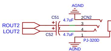
耳机输出电路
