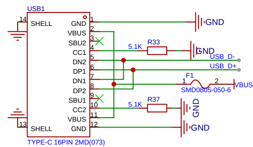
TYPEC接口
