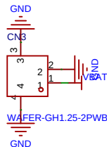
锂电池接口
