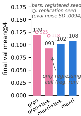
(d) GSM8K 2x2 (pre-registered)
