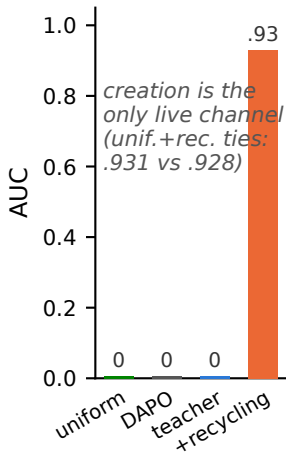
(b) Frontier ( p \leq 10^{-5} )
