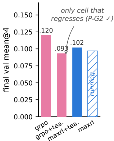
(d) GSM8K 2x2 (pre-registered)
