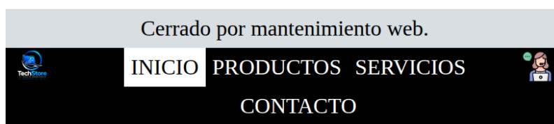
820 px de ancho con la fuente al 200 %: el menú salta a una segunda línea sin salirse de la cabecera.
