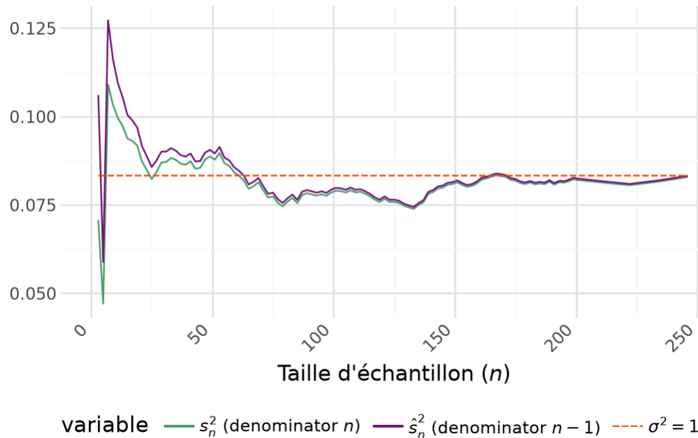
Figure 3. – Convergence de la variance empirique vers la variance théorique (question 3, Tip 1)
