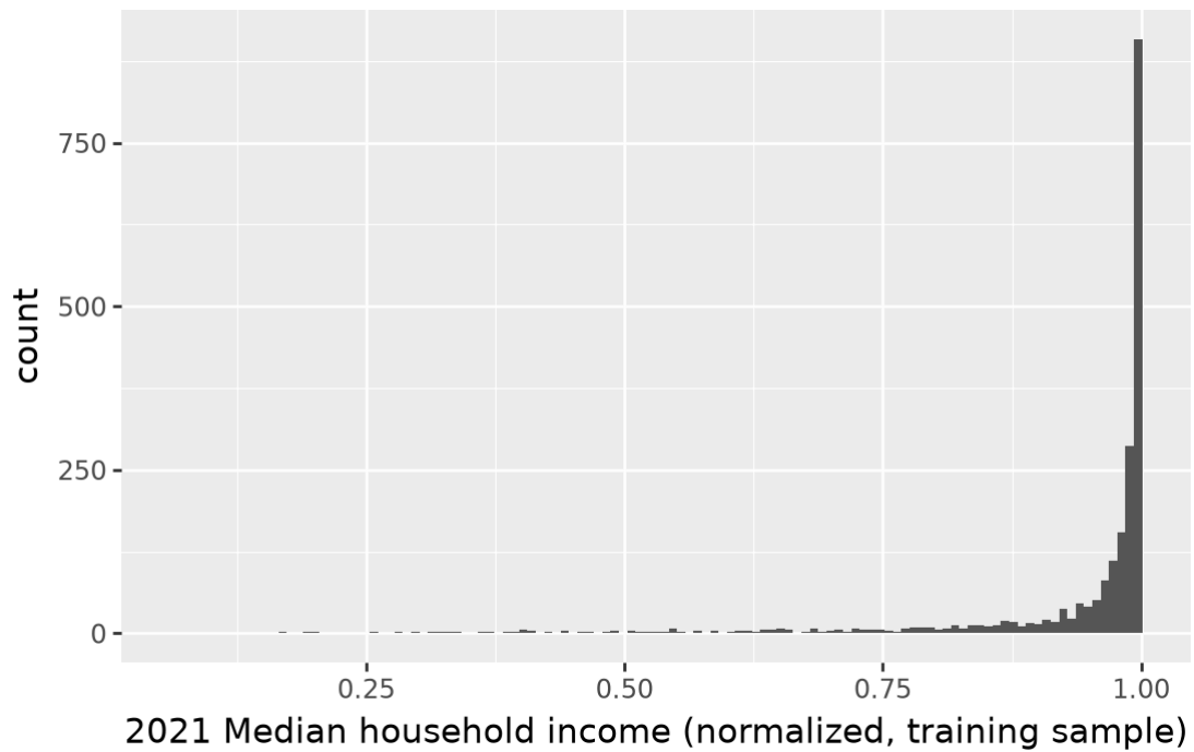
Figure 6. – Question 2, variable transformée, sur l'échantillon de normalisation
