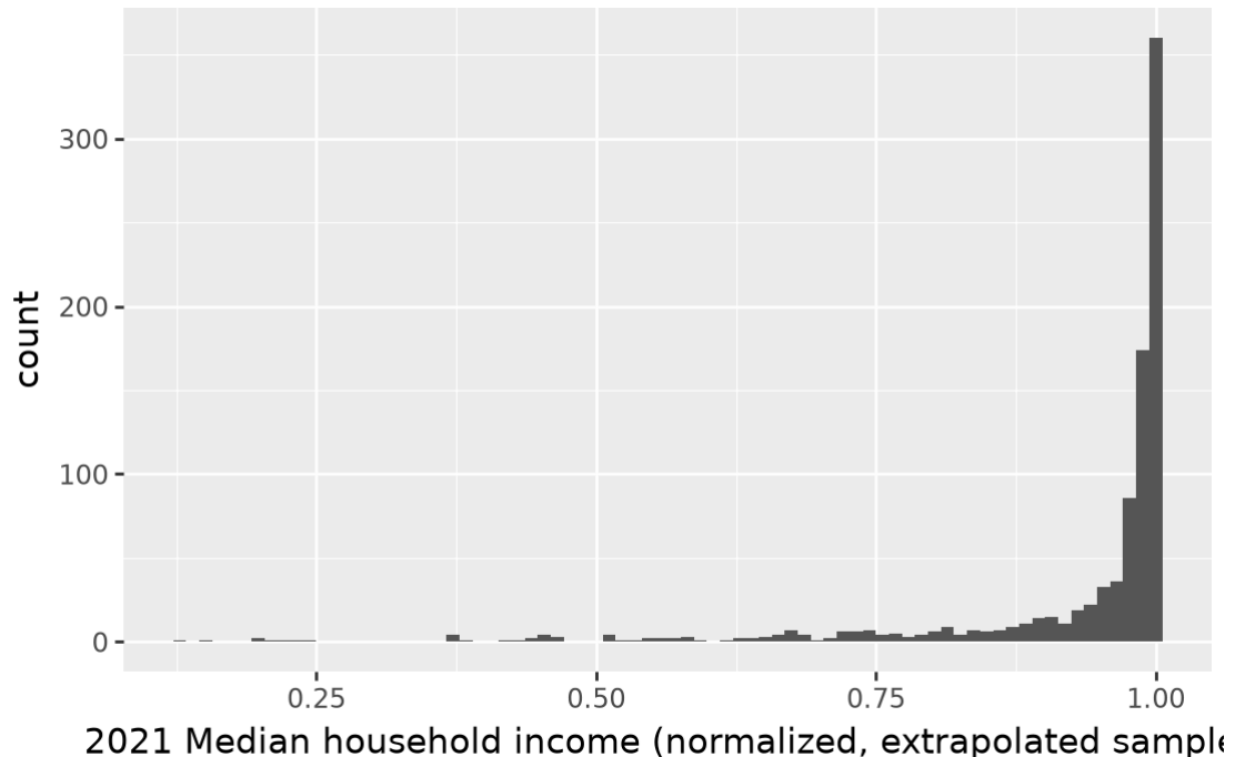
Figure 7. – Question 2, variable transformée, à partir des paramètres entraînés
