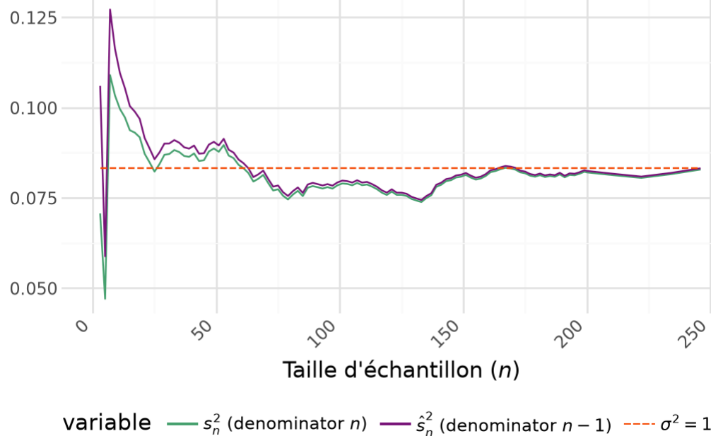
Figure 3. – Convergence de la variance empirique vers la variance théorique (question 3, Tip 1)
