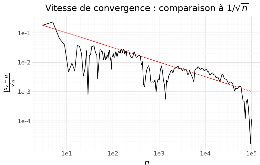
Figure 4. – Représentation de l'erreur d'estimation et son lien avec le nombre d'observations
