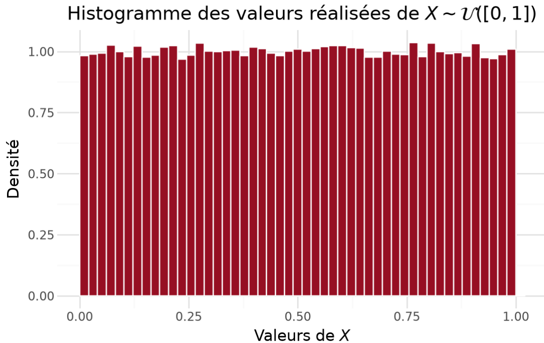
Figure 1. – Distribution empirique de notre tirage aléatoire de loi uniforme (question 2, Tip 1)
