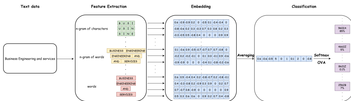
Figure 1. – Illustration de l'architecture de FastText
