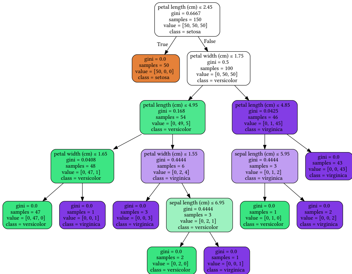
Figure 1. – Exemple d'arbre de décision sur le jeu de données classique iris. Source: Documentation de scikit-learn
