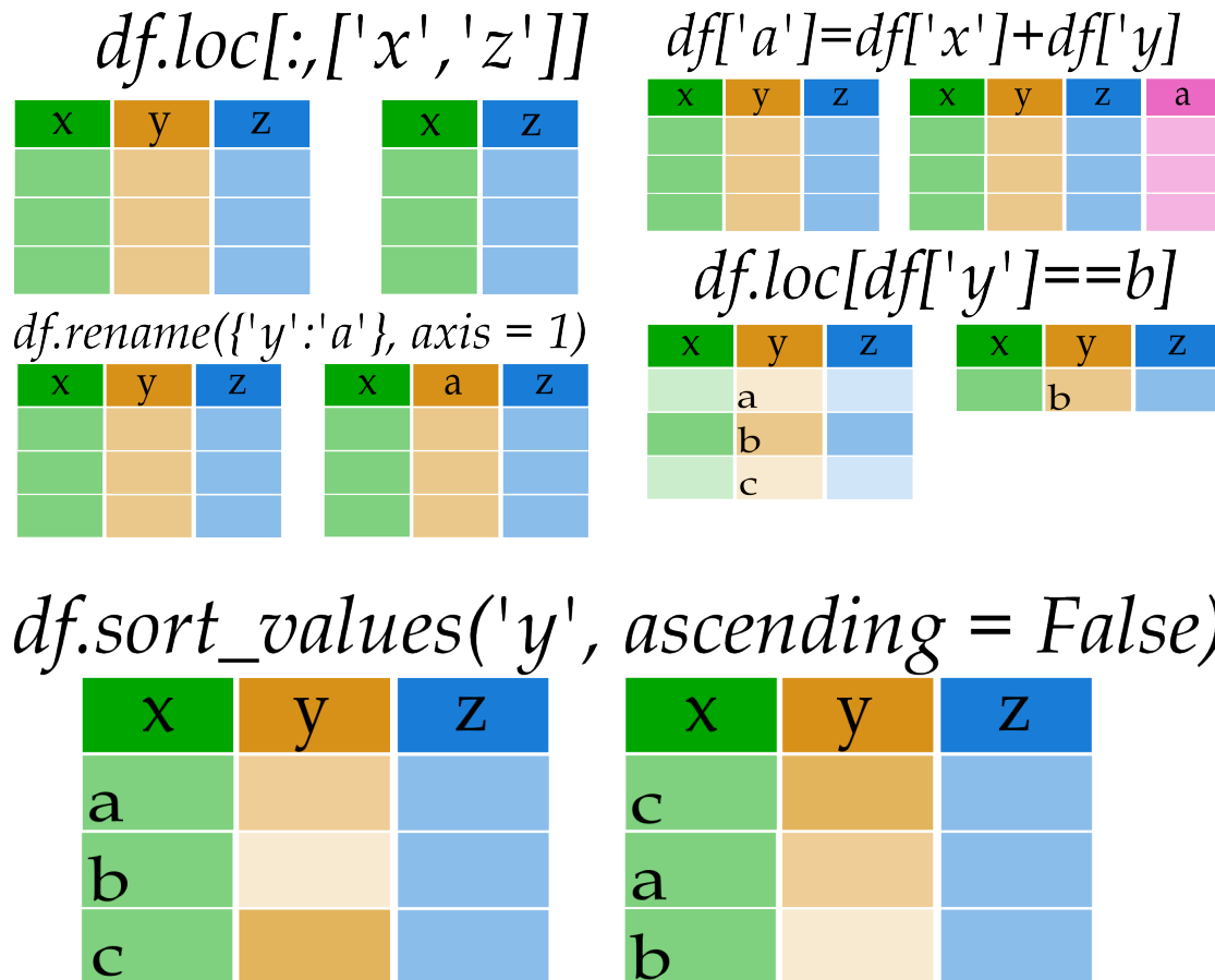
Fig. 1. – Réordonner le DataFrame
