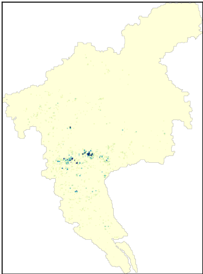
2015年 active_cnt 矩阵
