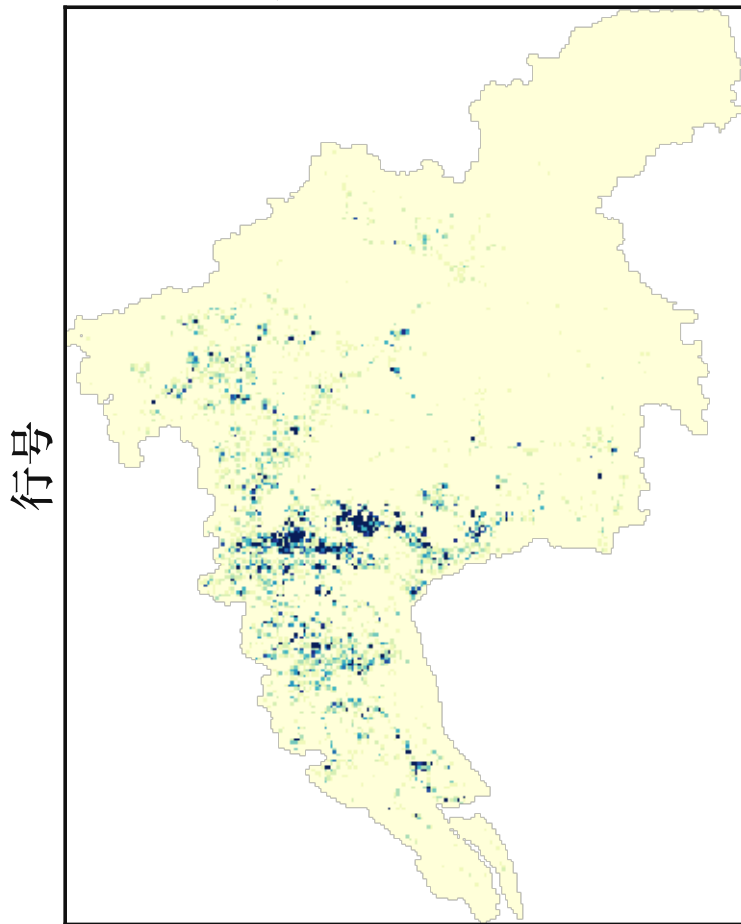
2024年 active_cnt 矩阵
