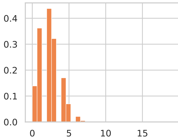
Baseline
