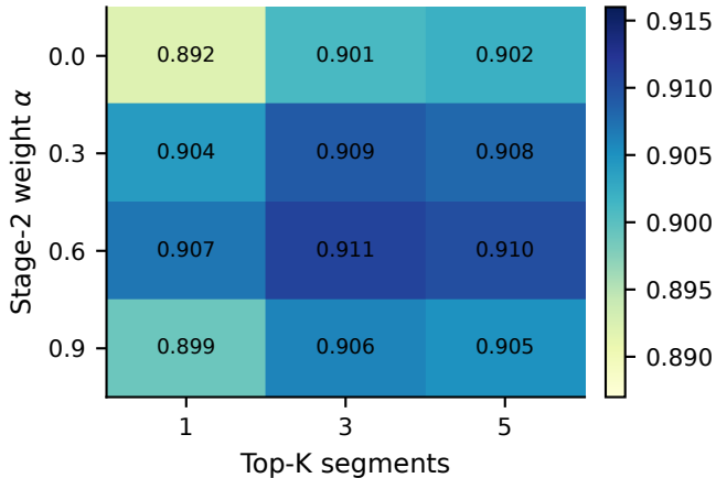
Macro-F1
