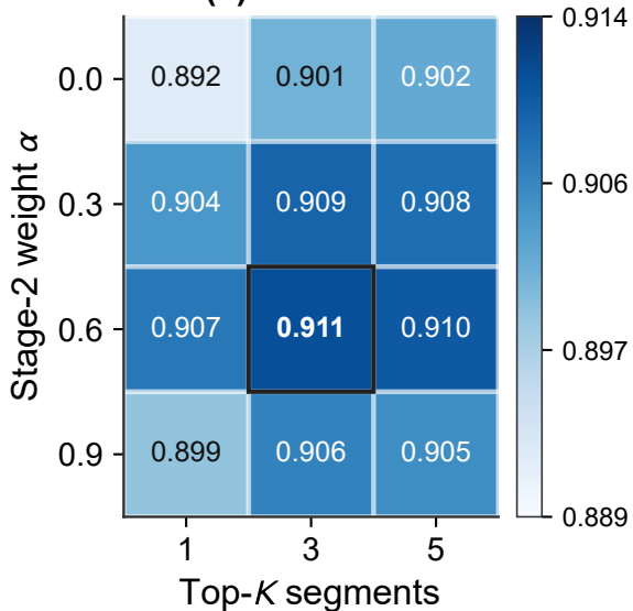
(a) Macro-F1
