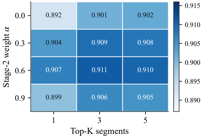
Macro-F1
