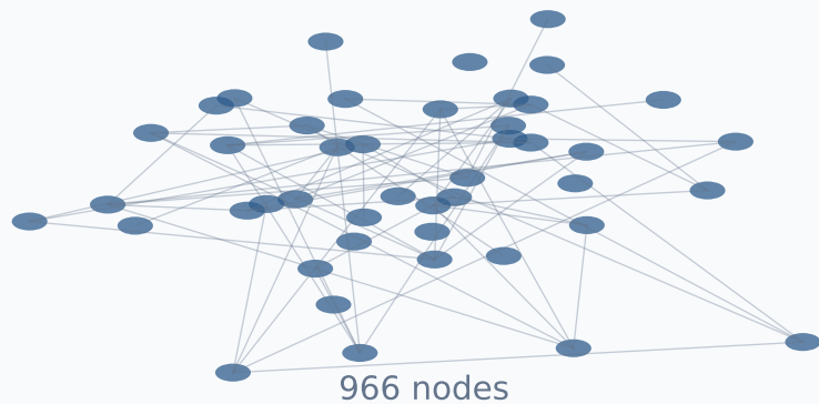
CNN
