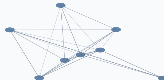
BiGRU
