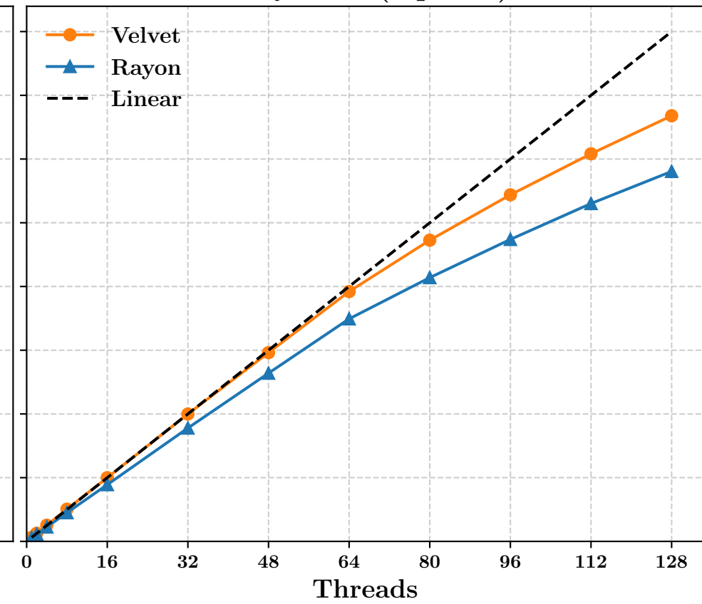
N-Queens ( nqueen )
