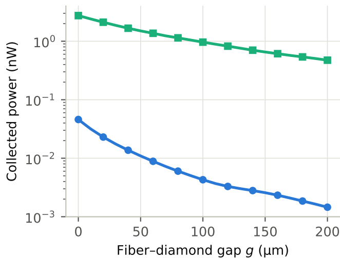
(d) ensemble, 10 mW exc.
