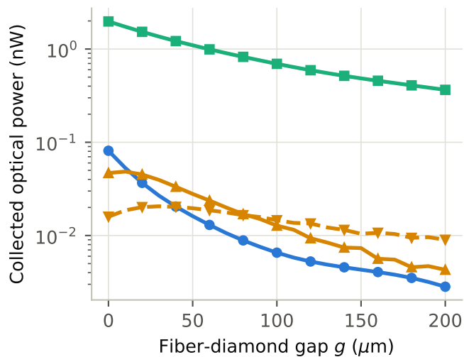
(d) 3D ensemble, 10 mW excitation
