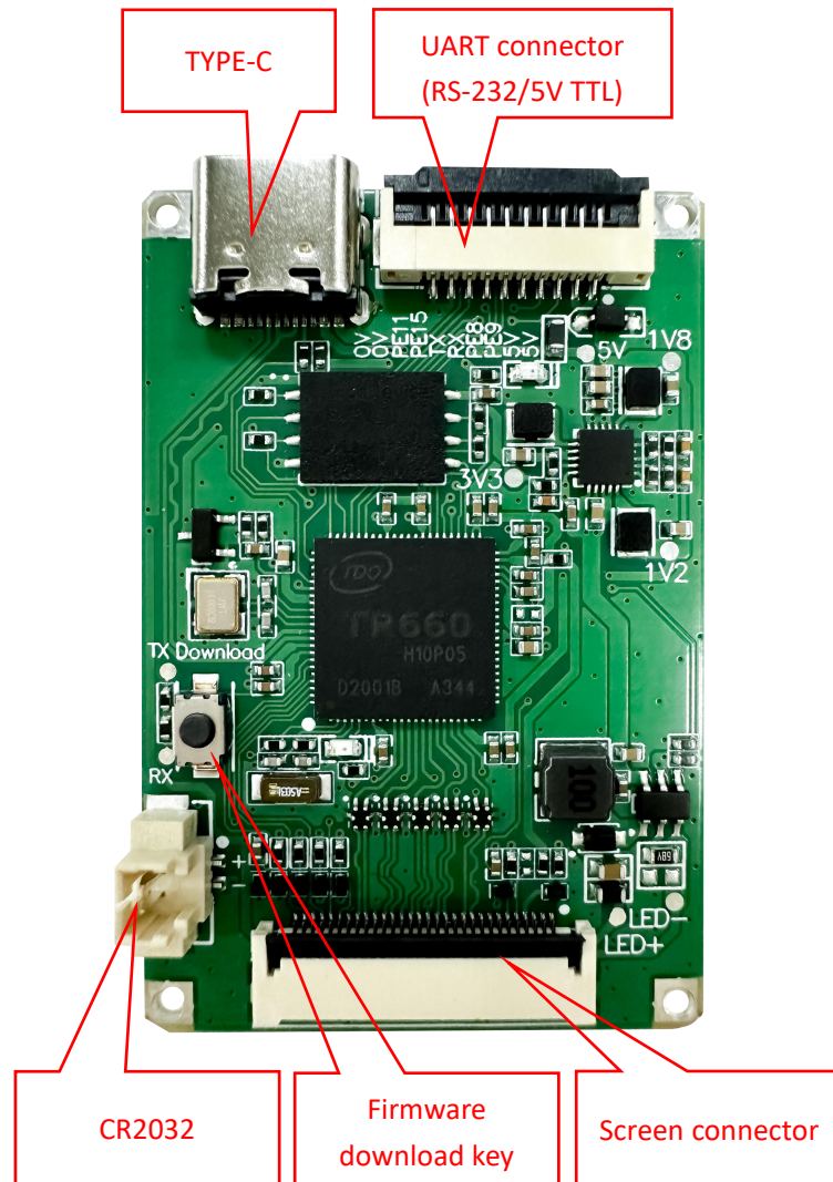
图 1.2-1 驱动板硬件配置参考图
