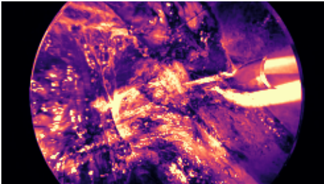
Retrieval error
