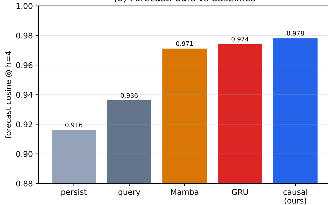
(d) Forecast: ours vs baselines
