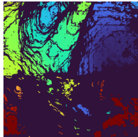
(d) Disparity
