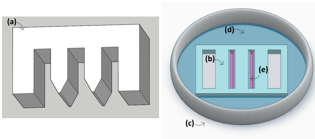
Figure 3: Dispositif expérimental pour les cultures quasi unidimensionnelles : vue 3D du moule imprimé en PETG (a) et schéma de la puce en PDMS intégrée dans une boîte de Pétri (b-e).
