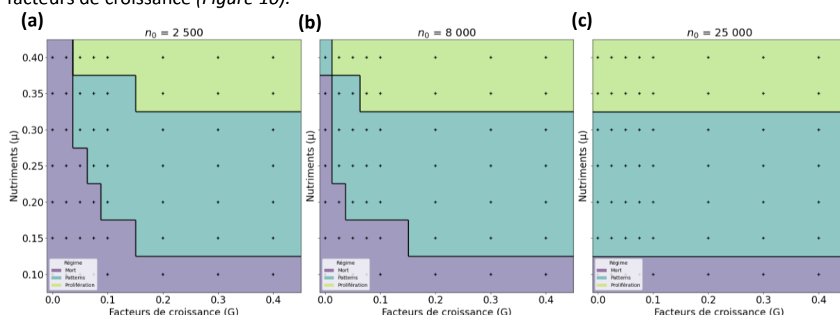
Figure 9 : Influence de la quantité cellulaire initiale sur le diagramme de phase : n_0 = 2\,500 cellules (a), n_0 = 8\,000 cellules (b) et n_0 = 25\,000 cellules (c), après 300 000h de simulation.
