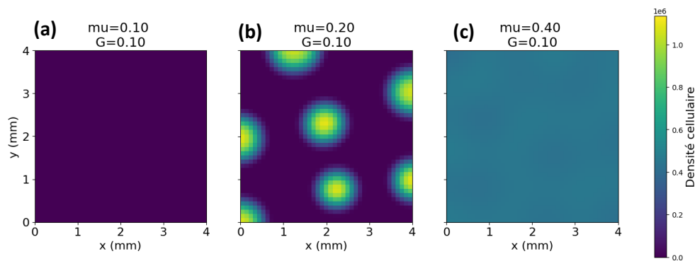
Figure 1 : Régimes dynamiques prédits par le modèle : disparition de la population cellulaire (a), émergence de motifs spatiaux (b) et prolifération homogène (c). Simulations réalisées avec 25 000 cellules initiales pendant 300 000 h.
