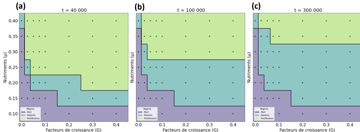
Figure 8 : Influence du temps de simulation sur le diagramme de phase : t = 40\,000\text{ h} (a), t = 100\,000\text{ h} (b) et t = 300\,000\text{ h} (c), avec 8000 cellules initiales.
