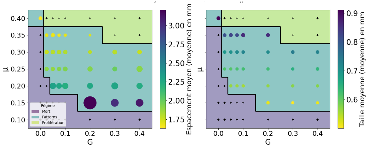
Figure 10 : Influence des conditions initiales sur les caractéristiques spatiales des motifs. Les couleurs représentent l'espacement moyen à gauche ou l'épaisseur moyenne des motifs à droite ; la taille des marqueurs indique la variabilité observée sur 20 simulations indépendantes. Simulations réalisées avec 8 000 cellules initiales pendant 300 000 h.
