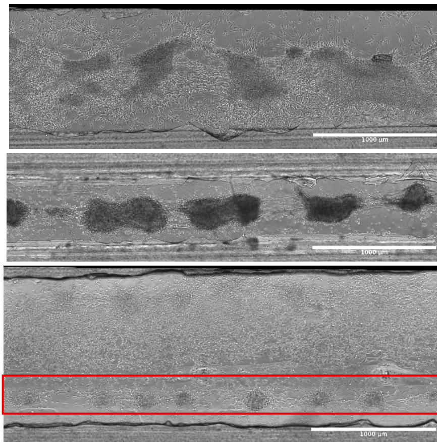
Figure 14 : Formation de motifs dans différentes géométries de puces unidimensionnelles. (a) Puce présentant une rainure de 1 \times 18 mm,ensemencée initialement avec 10 000 cellules et photographiée après 66 jours de culture. (b) Puce présentant une rainure de 0,5 \times 18 mm,ensemencée initialement avec 20 000 cellules et photographiée après 59 jours de culture. (c) Puce présentant une rainure de 1 \times 18 mm comprenant une zone de confinement d'environ 0,2 mm de largeur (zone indiquée en rouge),ensemencée initialement avec 40 000 cellules et photographiée après 19 jours de culture.
