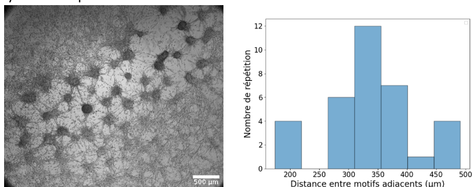
Figure 13 : Caractérisation spatiale des motifs obtenus pour la condition initiale \mu = 0,3 ; G = 0,03 au cours de l'expérience 2. À gauche : image des motifs observés. À droite : histogramme des distances entre motifs adjacents.
