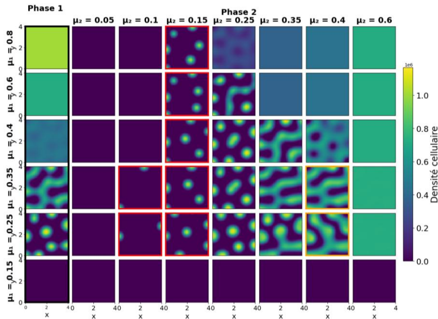
Figure 11 : Réversibilité des motifs après modification de la quantité de nutriment. La première colonne correspond à l'état obtenu après une phase initiale de simulation. Les colonnes suivantes montrent l'évolution du système après changement de la concentration en nutriments, mettant en évidence l'influence de l'état initial sur la dynamique finale. Les zones entourées en rouge correspondent à des conditions où des motifs persistent alors qu'elles auraient initialement mené à la mort. Les zones entourées en orange correspondent à des conditions où les motifs persistent alors qu'elles auraient initialement mené à de la prolifération. Simulations réalisées avec G = 0,03 et 25 000 cellules initiales pendant 300 000 h.
