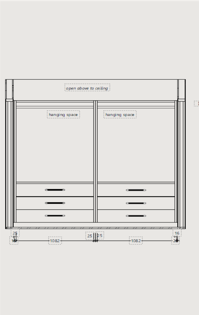
ELEVATION
