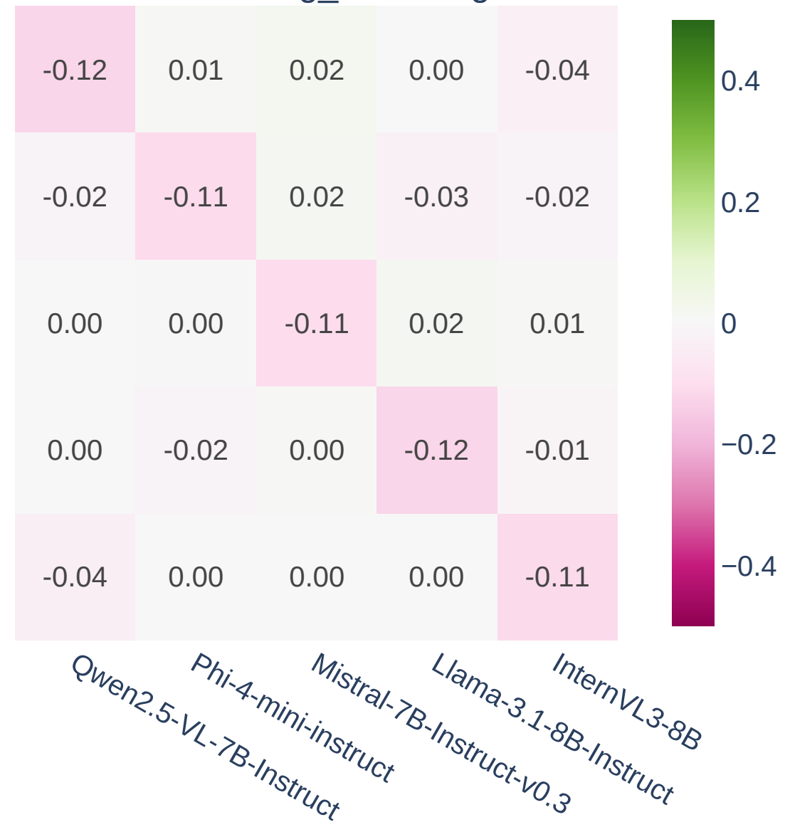
embedding_clustering
