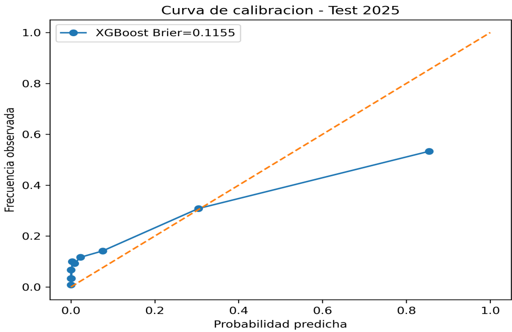
Figura 5: Curva de calibracion - Test 2025
