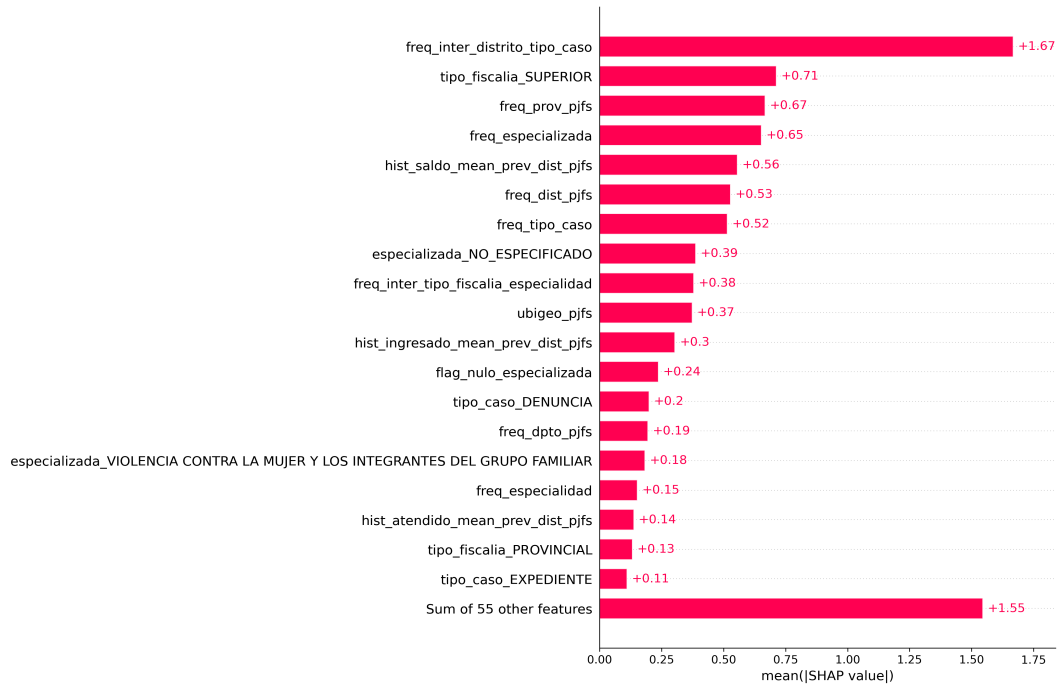
Figura 2: SHAP Bar Chart - Importancia media absoluta
