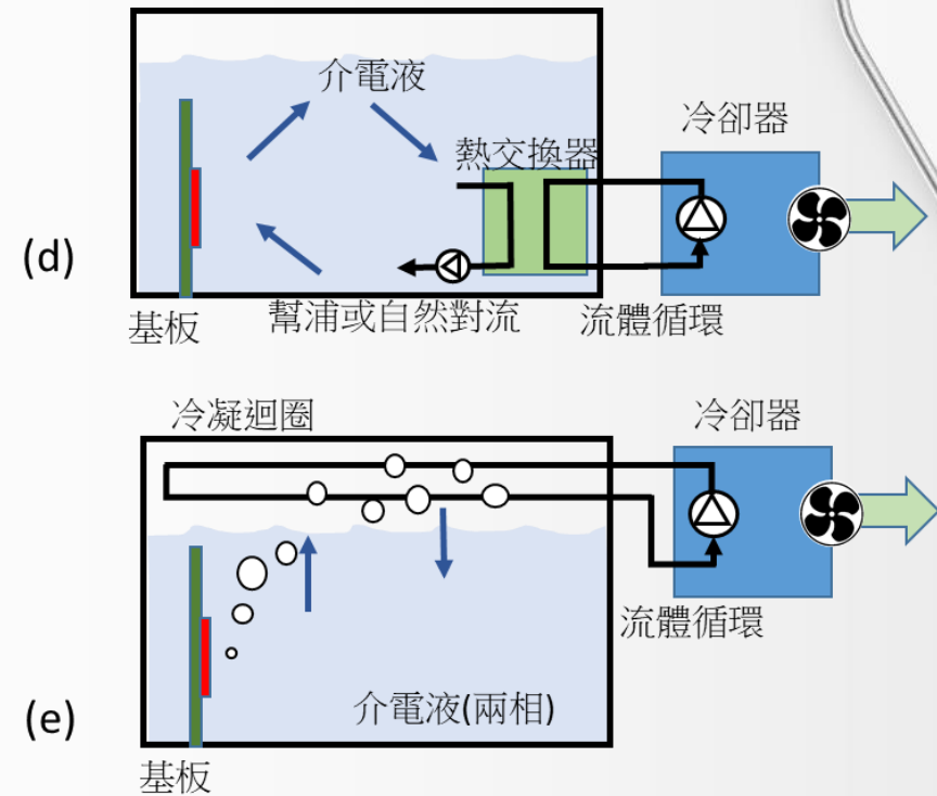
(a)直接至晶片冷卻單相液冷 (b)直接至晶片冷卻雙相液冷 (c)浸沒式機殼型式單相及雙相液冷 (d)浸沒式管型式單相液冷 (e)浸沒式管型式雙相液冷
