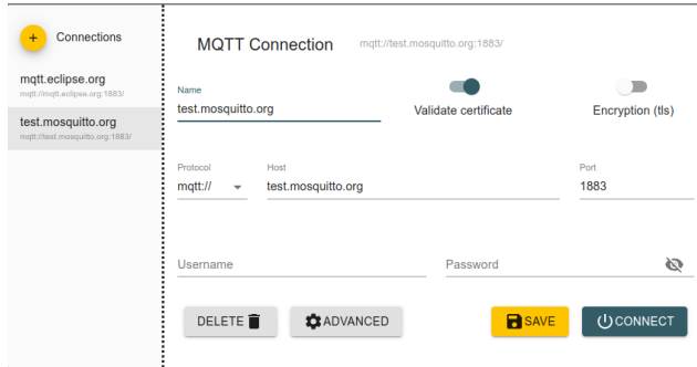
Figure 8: Verbindung MQTT Explorer mit testMosquitto Broker
