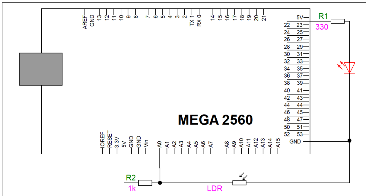
Abbildung 1: Schaltplan
