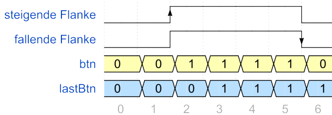
Figure 10: Werte der Variablen btn und lastBtn
