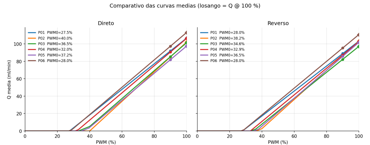
Figura 5: As seis curvas médias. Losango: Q_{100} .
