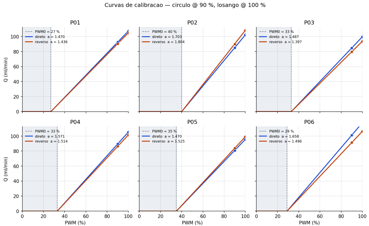
Figura 1: Rodada 1: Q = 0 até PWM_0 . Círculo: Q medido @ 90 %. Losango: Q_{100} do modelo.
