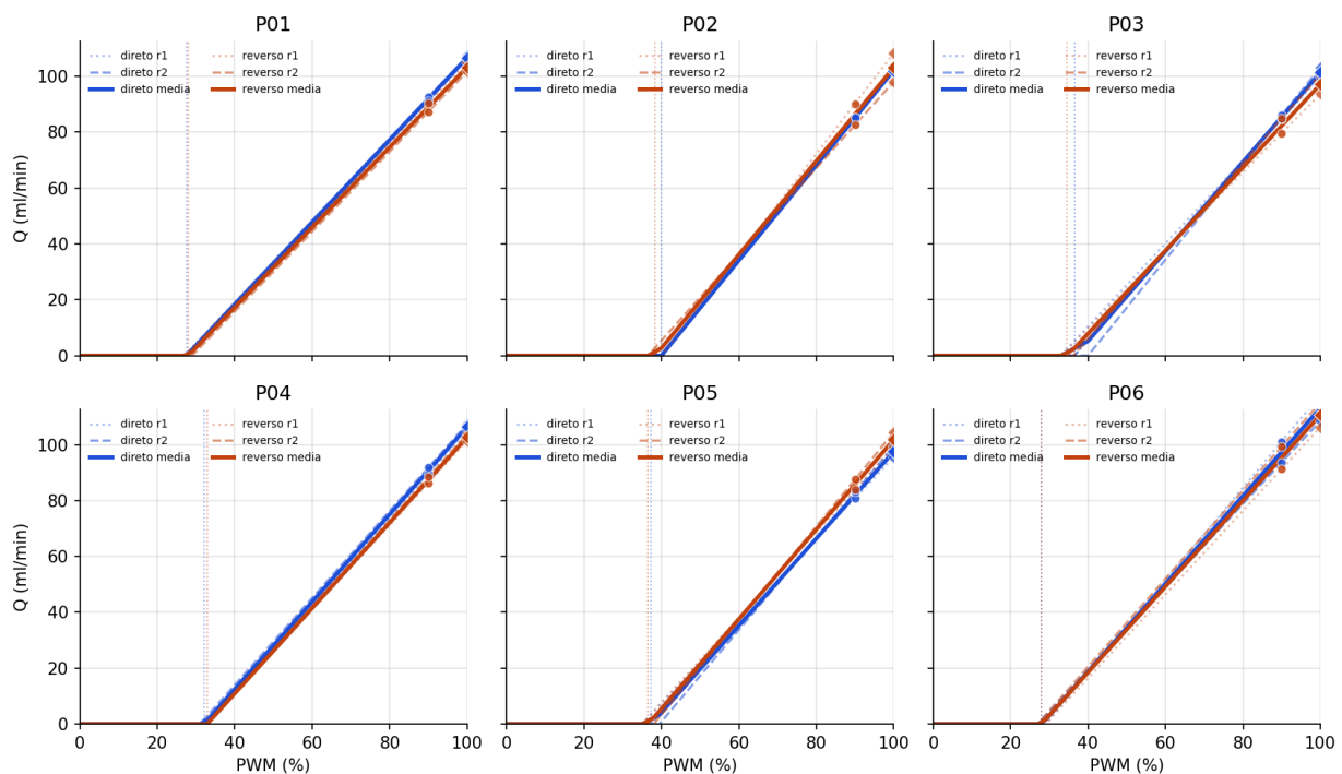
Figura 4: Curvas das duas rodadas e a média. Círculo @ 90 % (medido); losango @ 100 % (modelo).
