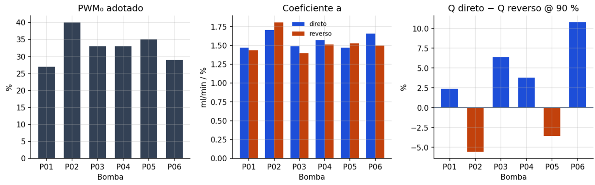
Figura 3: Rodada 1: PWM_0 adotado, coeficiente a e assimetria direto/reverso @ 90 %.
