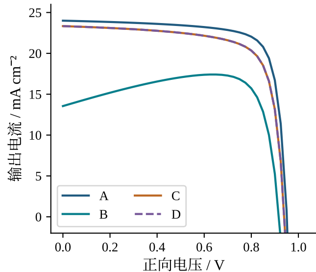
光伏工作区
