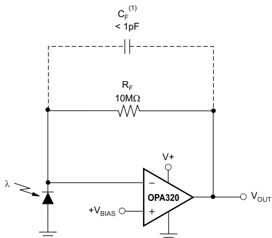
图 41. 单电源跨导放大器
