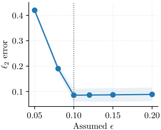
Error
