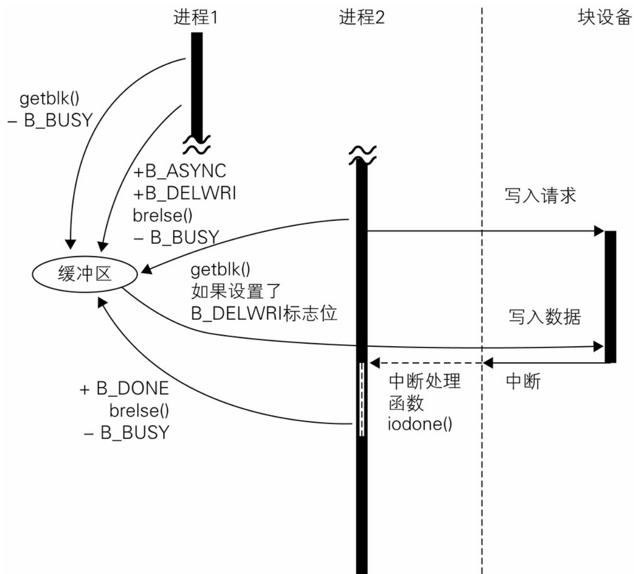
图 7-11 延迟写入
