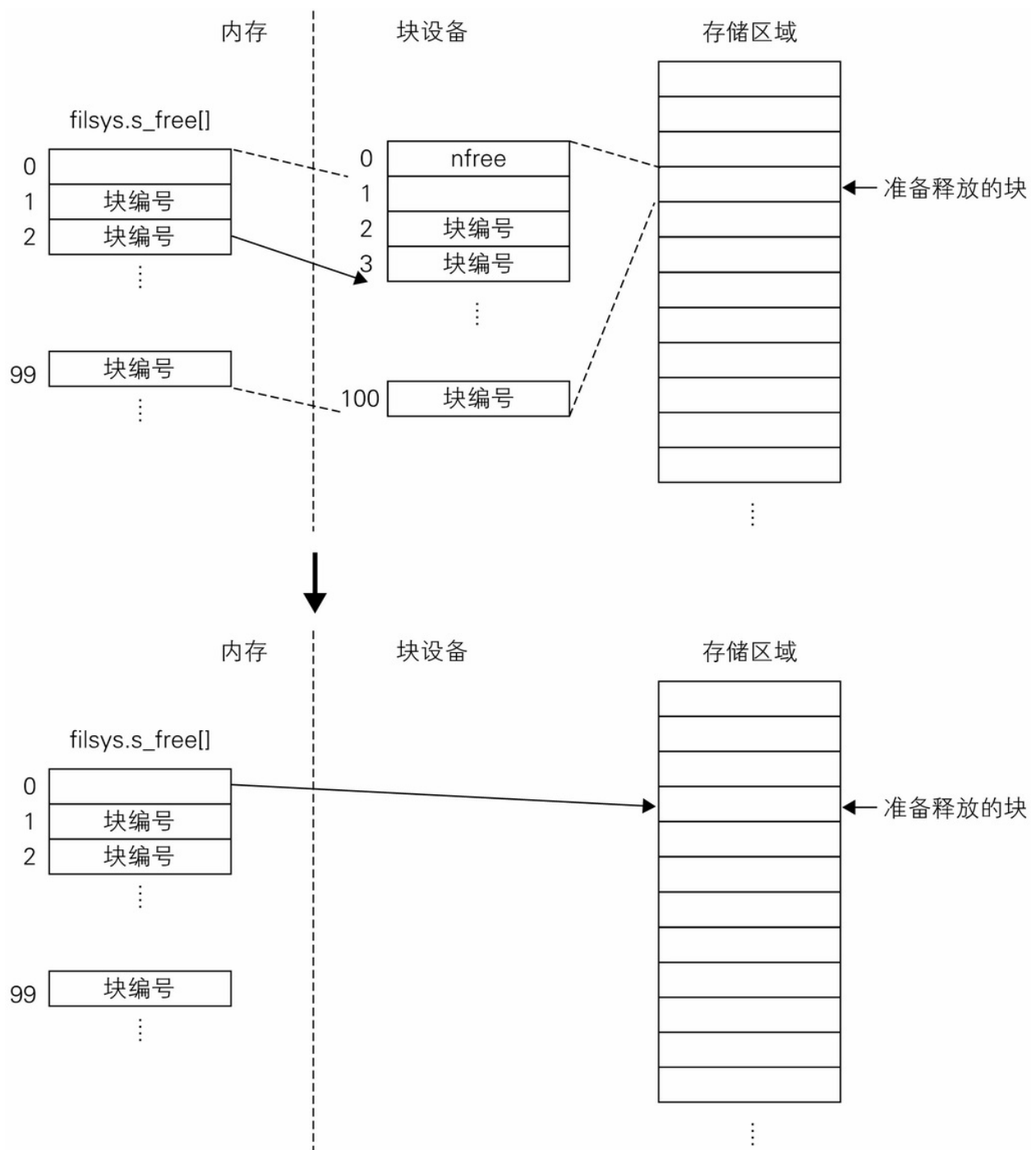
图 9-15 free()
