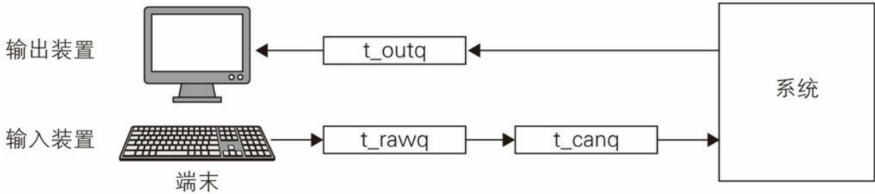
图 13-4 3 个缓冲区
