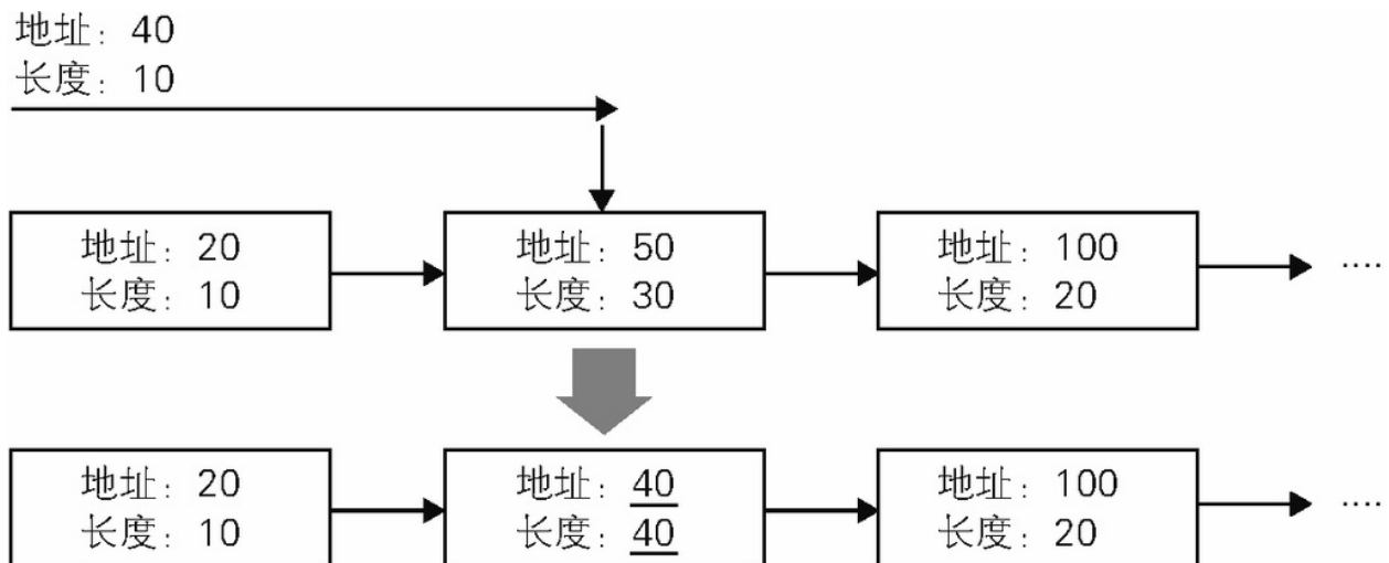
图 3-27 区域的合并
