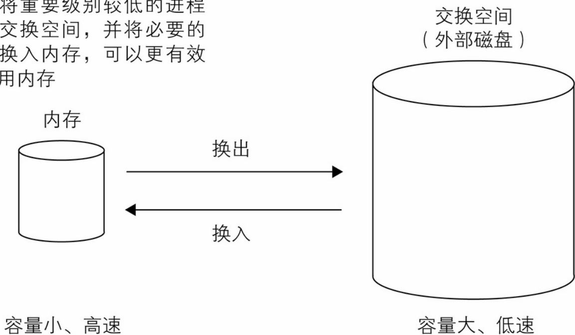
图 4-1 交换处理
