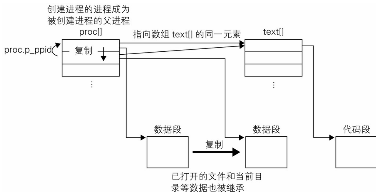
图 3-2 进程的生成
