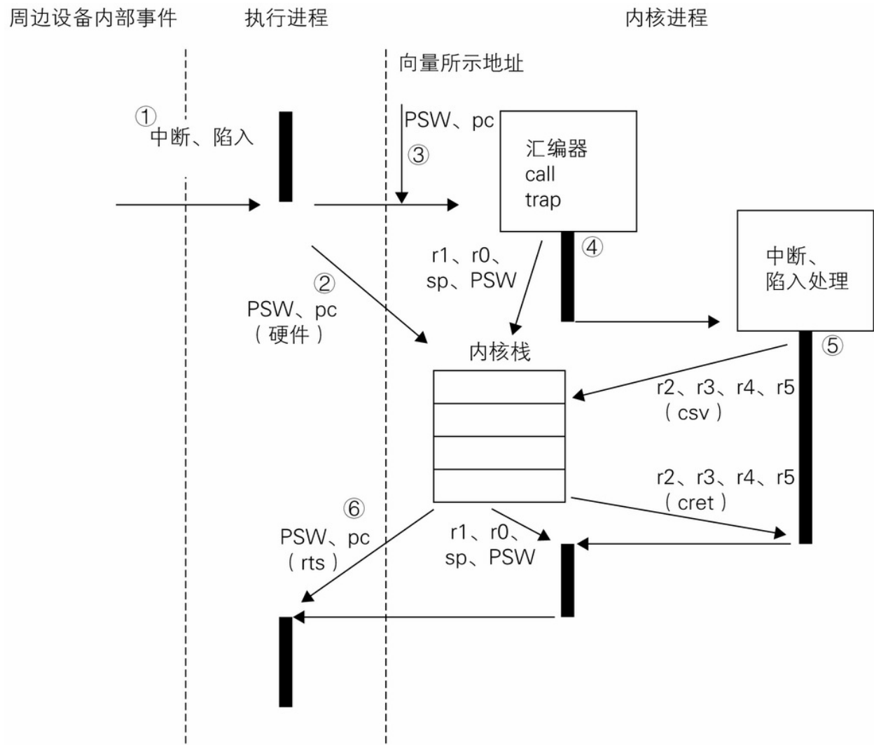
图 5-5 中断和陷入
