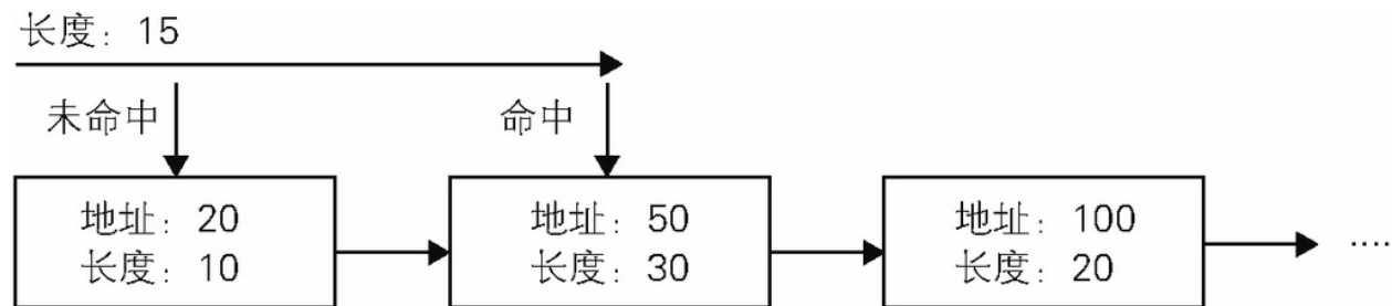
图 3-22 First Fit
