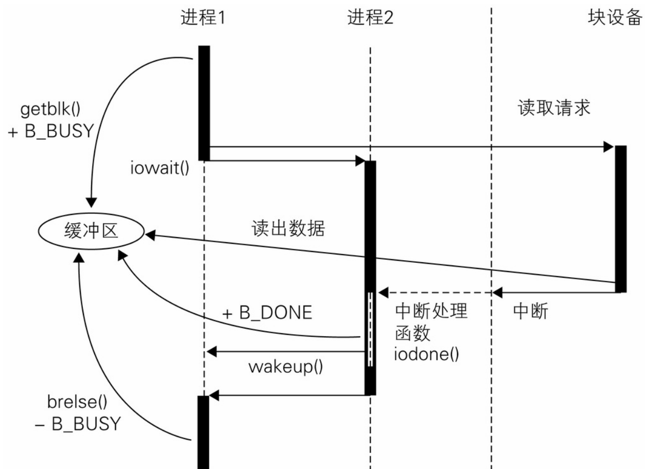
图 7-9 同步读取
