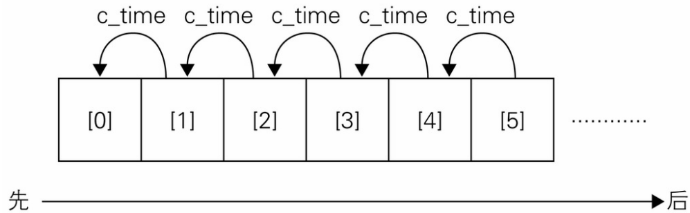
图 5-7 callout[]
