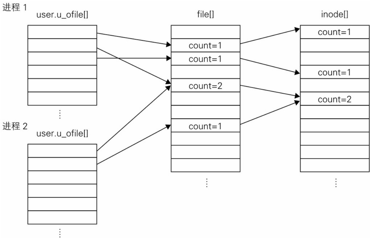
图 10-1 打开文件
