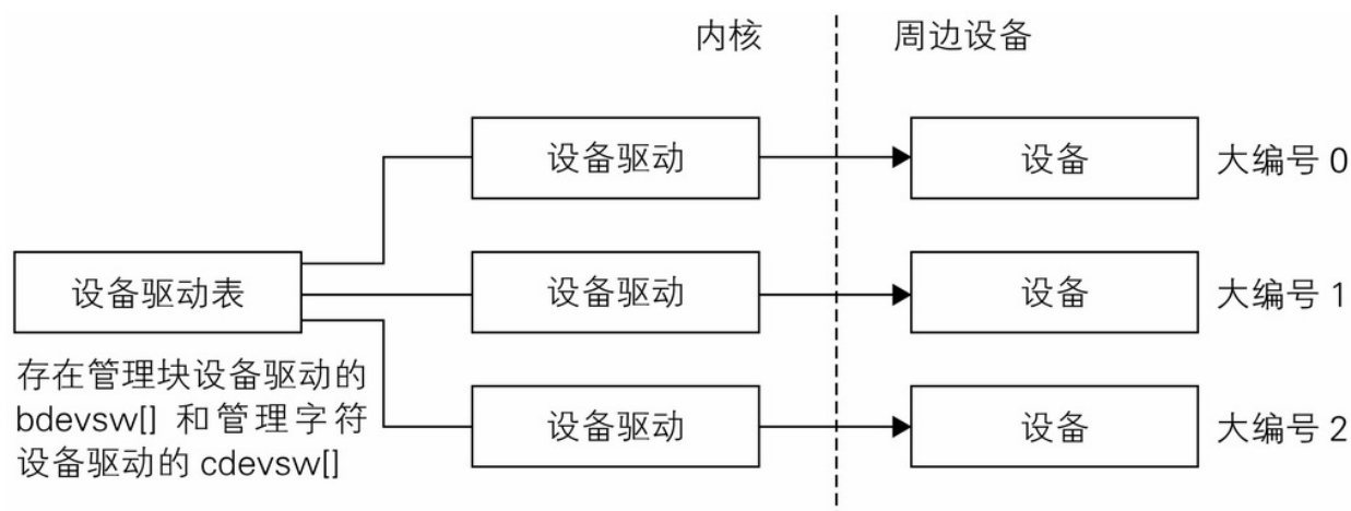
图 7-1 设备驱动表
