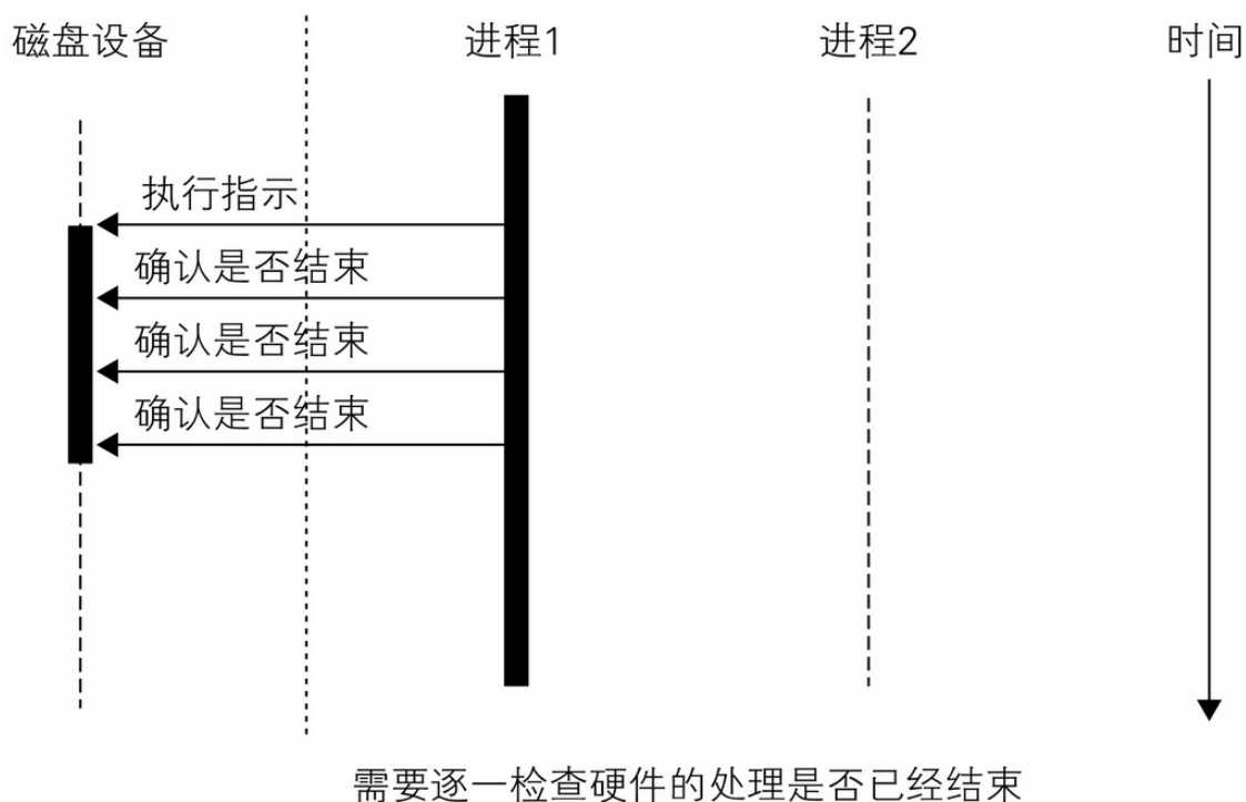
图 5-2 轮询
