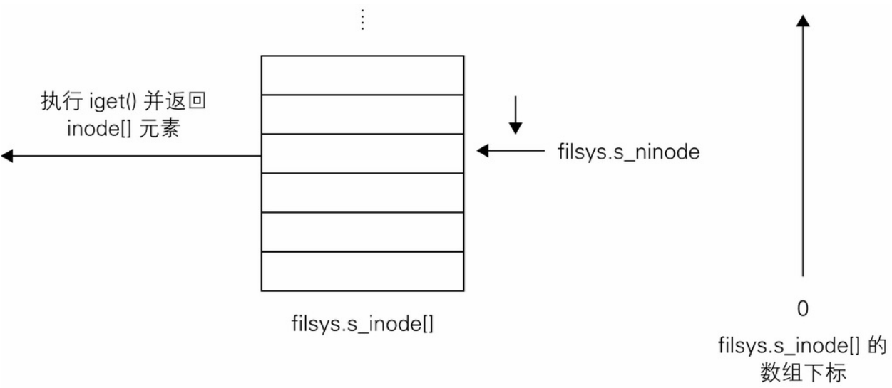
图 9-10 ialloc()
