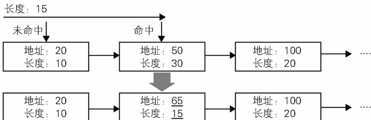
图 3-23 命中
