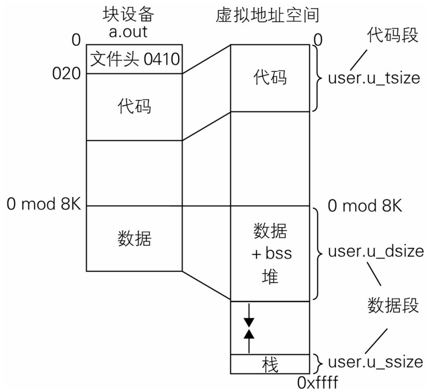
图 3-12 魔术数字 0410
