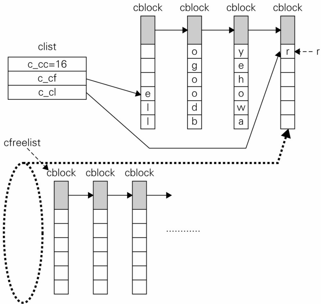
图 12-5 putc()
