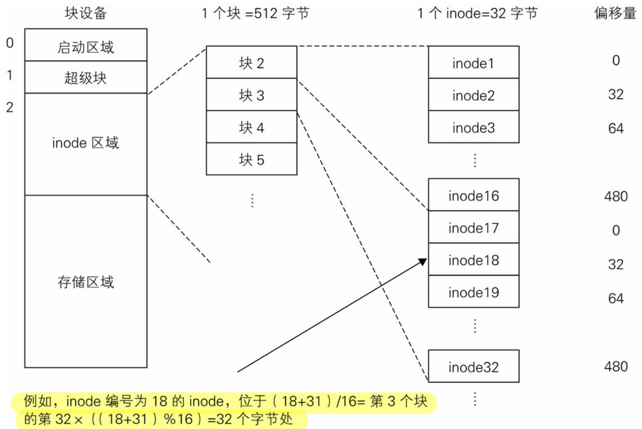
图 9-4 inode 区域
