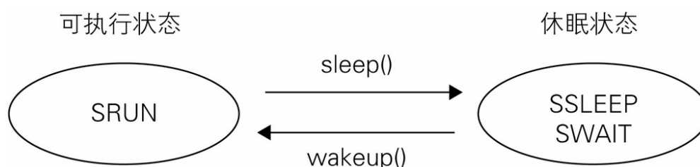
图 3-7 状态迁移图
