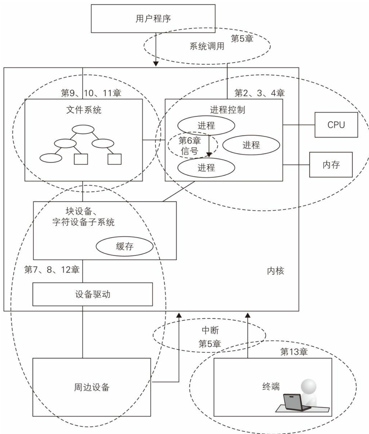
图 1 内核整体结
