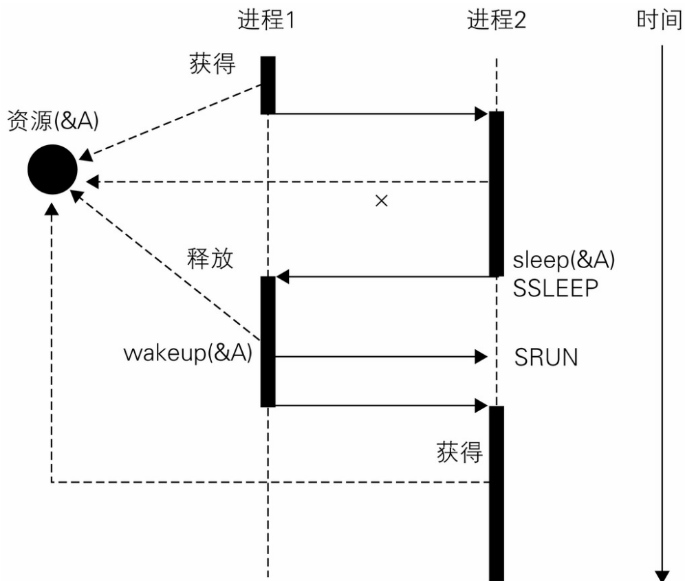
图 3-8 sleep() 和 wakeup()
