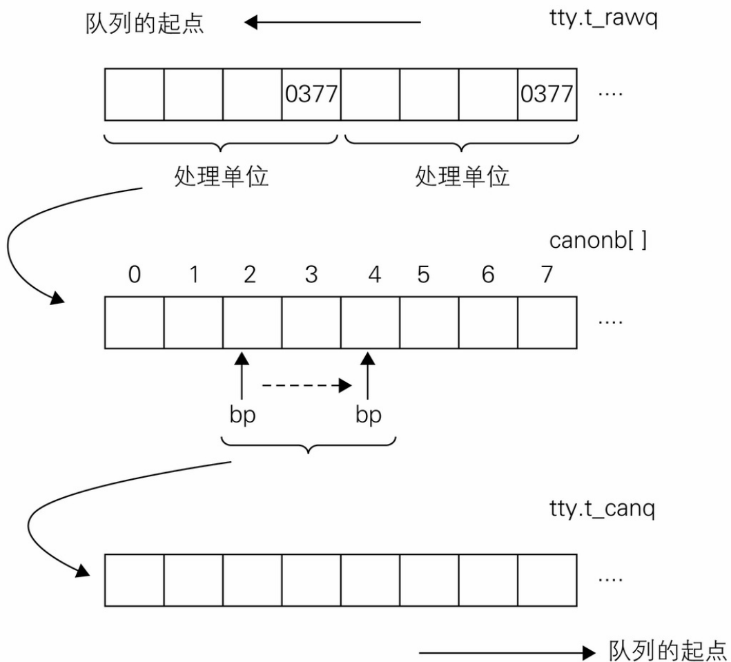
图 13-8 canon()
