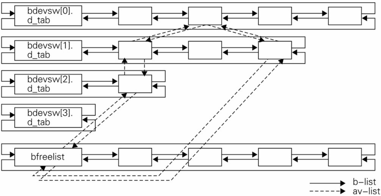
图 7-6 b-list 和 av-list
