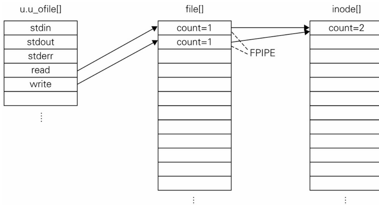
图 11-2 pipe()
