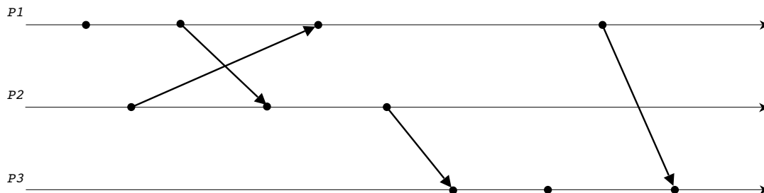
FIG. 1 – Exécution de l'algorithme de Singhal et Kshemkalyani
