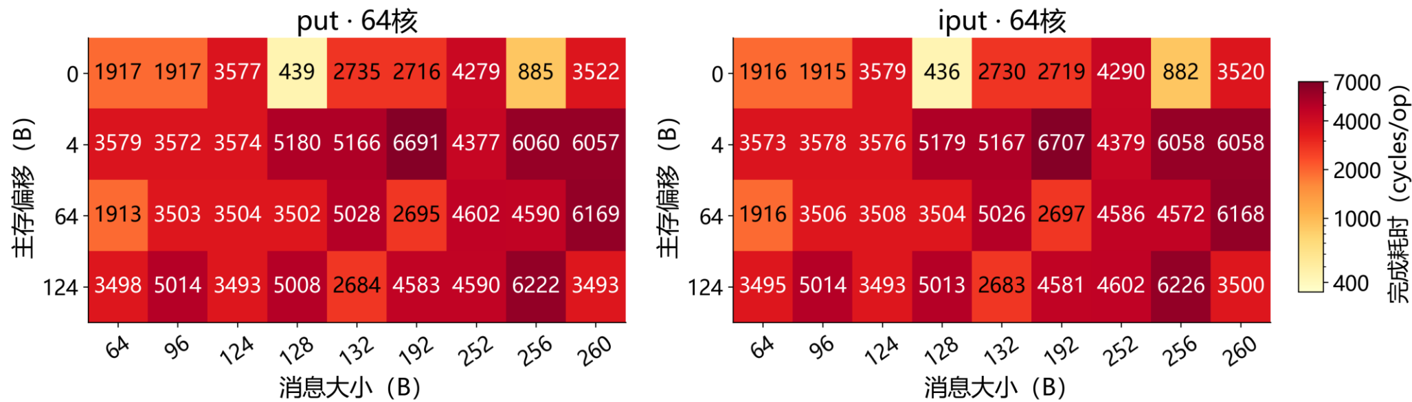
图 6 64 核 put 与 iput 完成耗时 格内数值为 cycles/op，四舍五入到整数；色标仅适用本页
