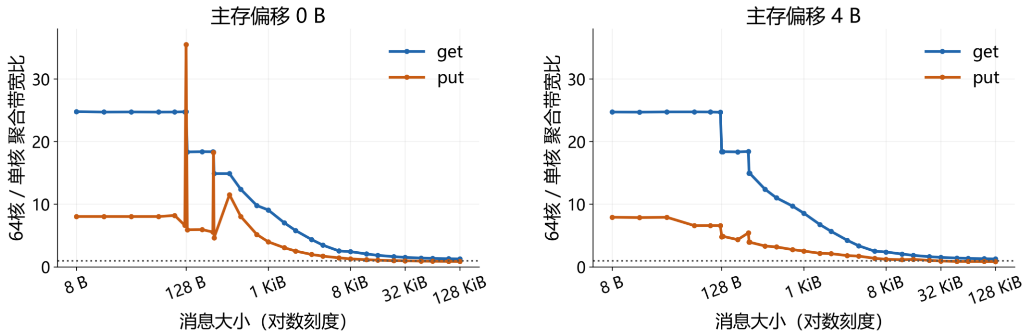
图 3 64 核相对单核的带宽收益 左为偏移 0 B，右为偏移 4 B
