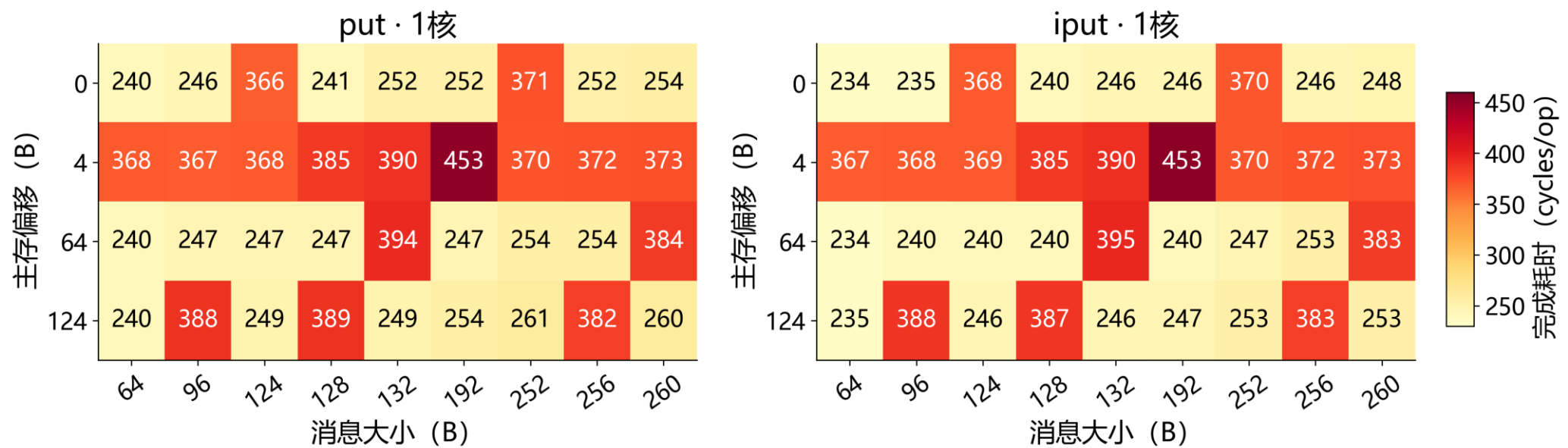
图 5 1 核 put 与 iput 完成耗时 格内数值为 cycles/op，四舍五入到整数；色标仅适用本页
