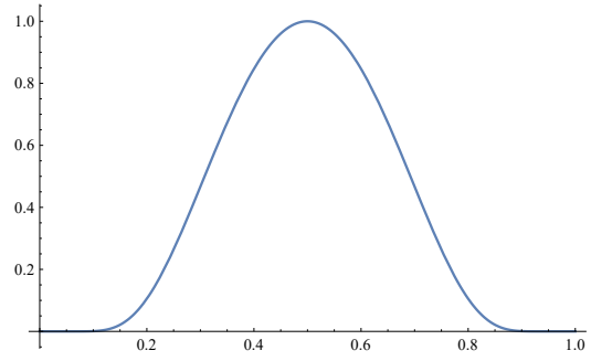
图 4.3: 指数函数积 g
