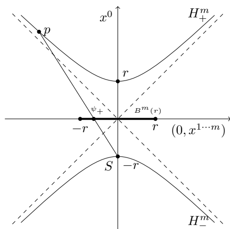
图 10.1: 双曲空间
