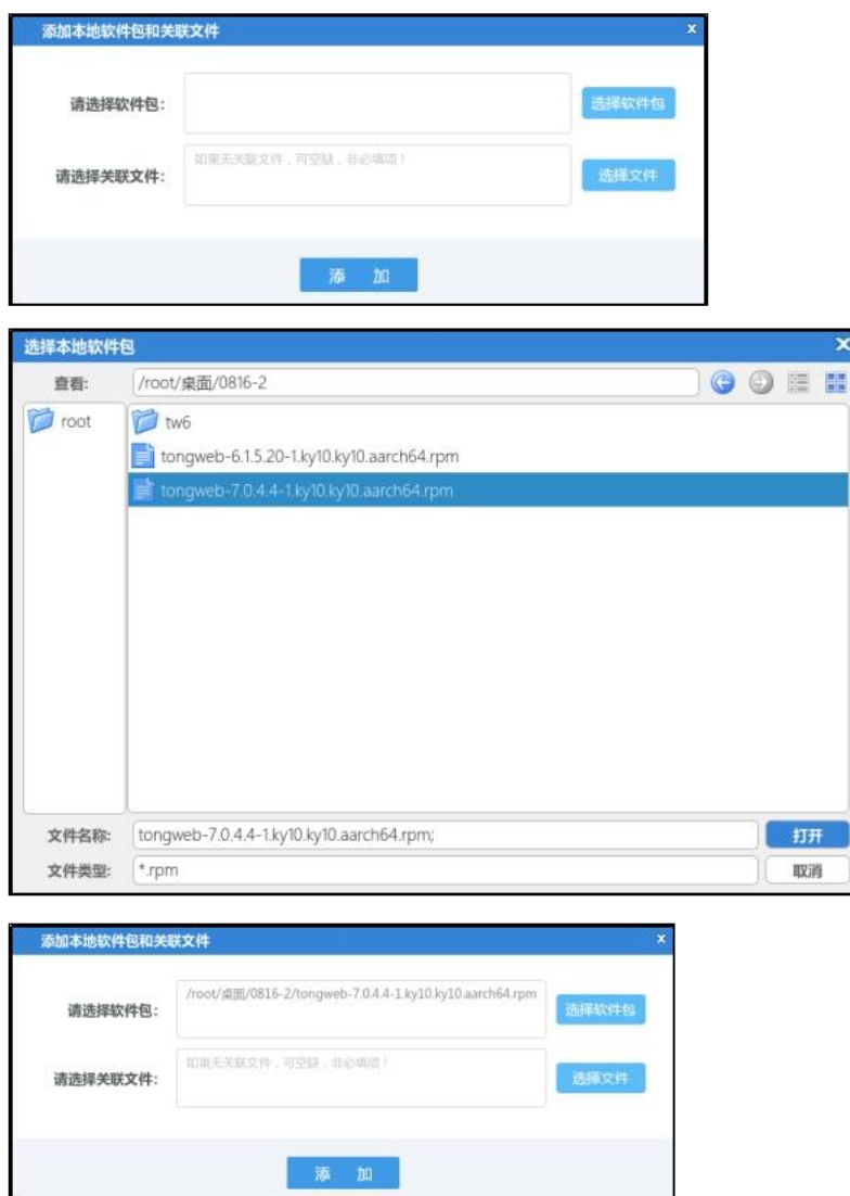
图 2.3-2：选择安装软件包
