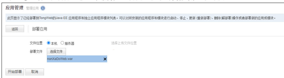
图 3.3-1：部署应用
