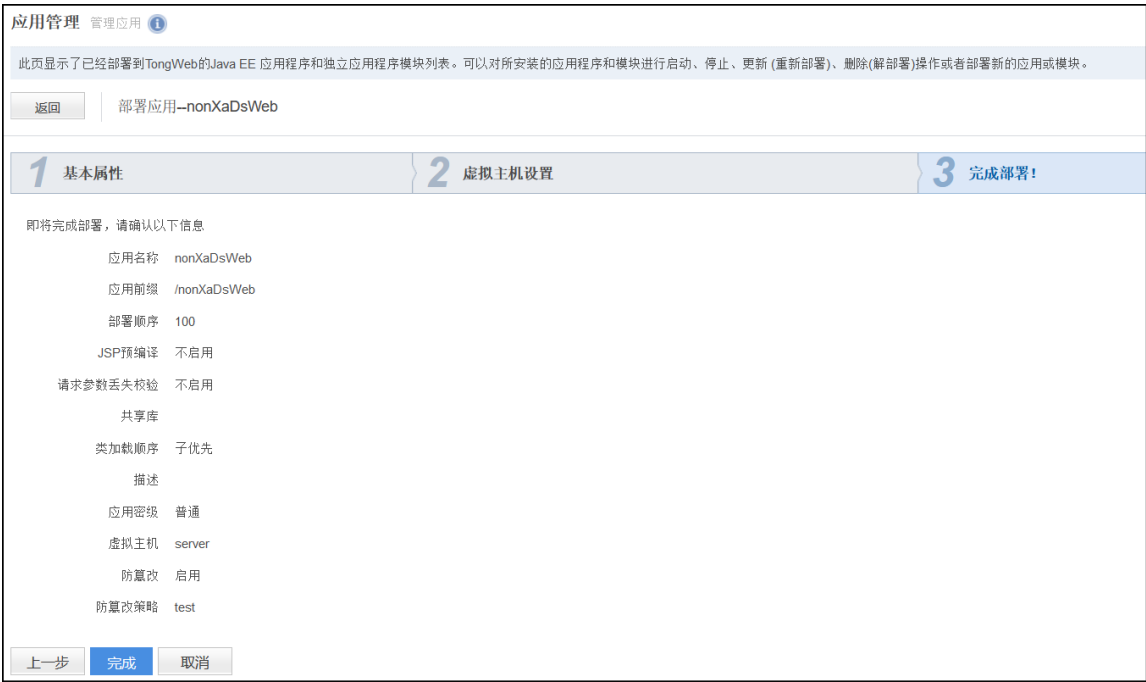
图 3.3-4：部署应用-部署完成
