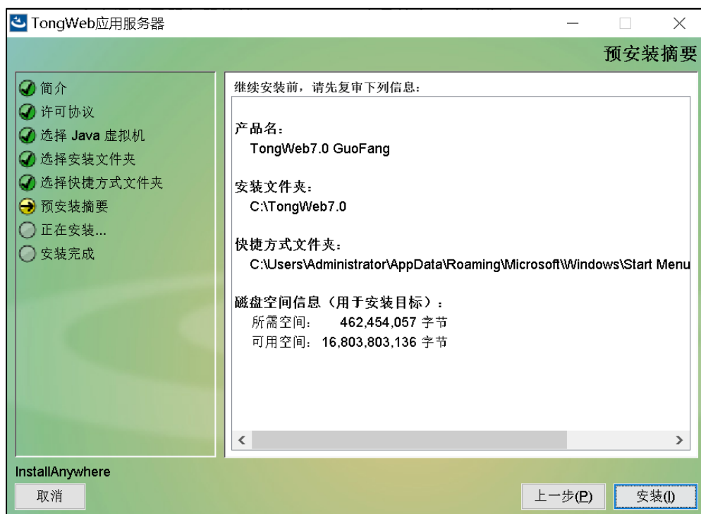
图 2.3-7：预安装界面
