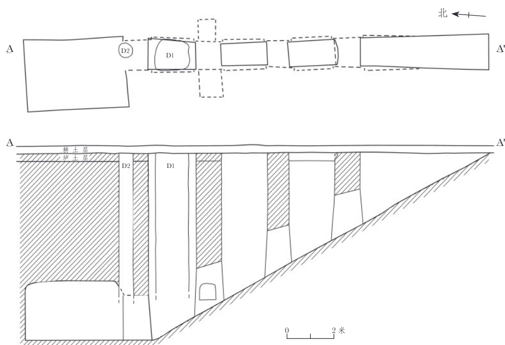
图三 M2338 平、剖面图
