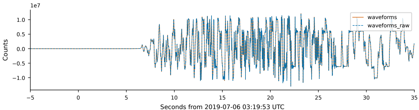
b Gap handling · CI.WBP HHE
