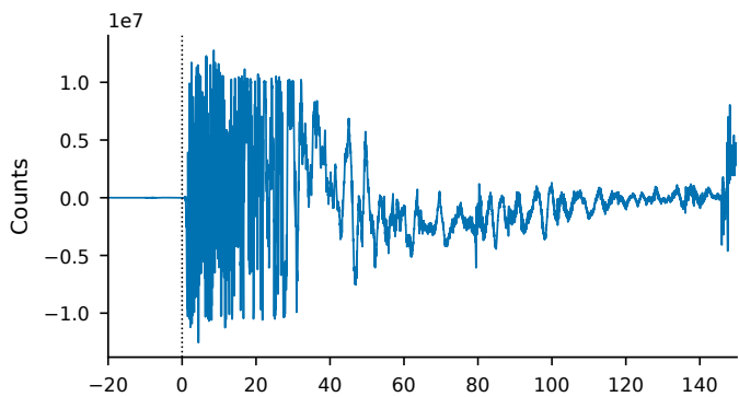
f PB.B918 EH Z · Mw 7.1
