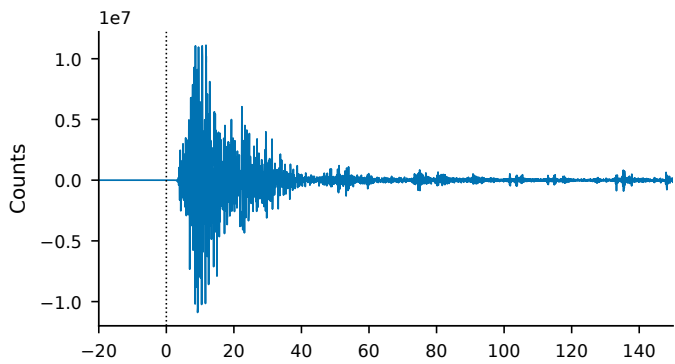
f PB.B918 EH Z · Mw 7.1
