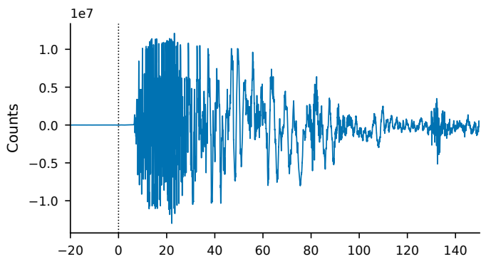
d Cl.CLC HHZ · Mw 7.1
