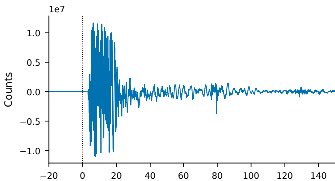
e PB.B918 EH Z · Mw 6.4
