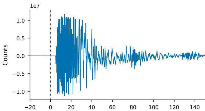
c Cl.CLC HHZ · Mw 6.4
