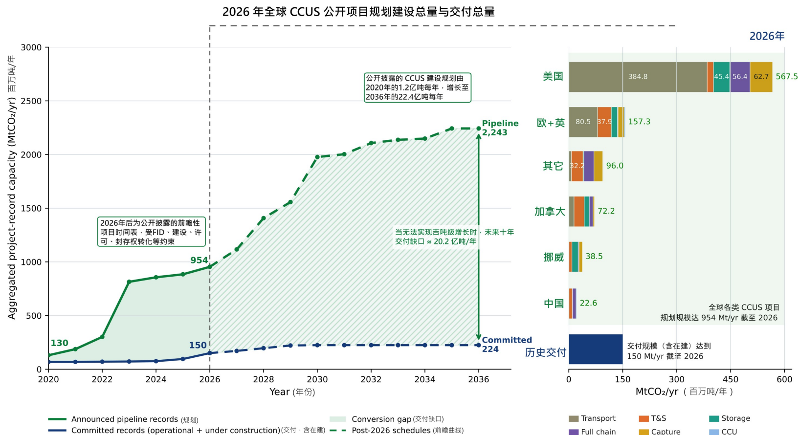
图1 全球 CCUS 前瞻性项目规划与已进入工程实施阶段记录规模的转化差距 (2020–2036)
